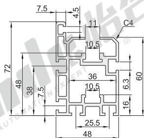
ATS05-30-31DG (此型号需另外采购钢轨)
