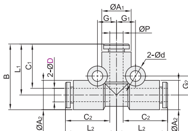
T型三通接头 XZR43
