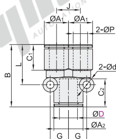
Y型三通接头 XZR42
