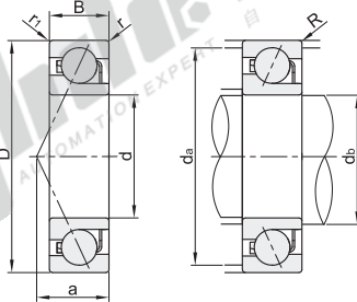
■ 安装图
