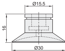
盘径Ø30
