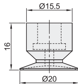
盘径Ø20
