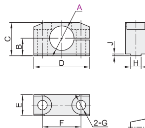
圆孔型 BWA10
