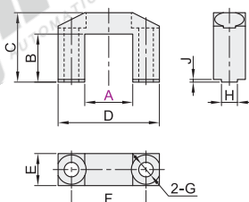
方槽型 BWA09
