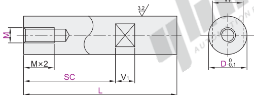
一端内螺纹型 RAC01/02/03/06
