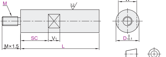
一端外螺纹型 RAC11/12/13/16
