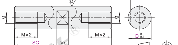
带扳手槽型 RAD11/12/13/16/18
