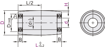
圆弧型 ENL61/71/81/86
