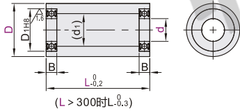
直柱型 ENL01/11/21/26
