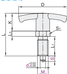
自锁型 无锁紧螺帽 ZAU40/46
