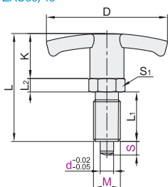
复位型 无锁紧螺帽 ZAU39/45
