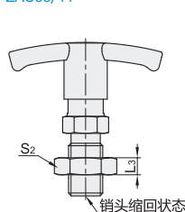
带锁紧螺帽 ZAU38/44
