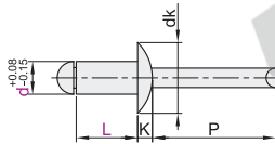
开口型平圆头 TBC61/64
