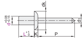
封闭型扁圆头 TBC65/66
