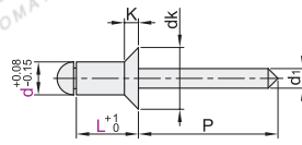
开口型沉头 TBC62/63
