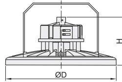
安装方式：2(框架安装)
