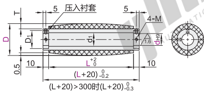
圆孔+螺孔型
