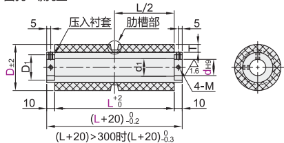
圆孔+螺孔型
