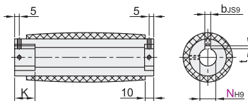
键槽孔+螺孔型
