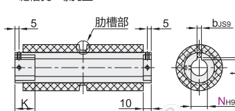
键槽孔+螺孔型
