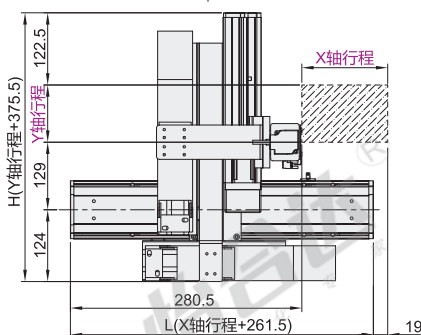
● X轴尺寸
