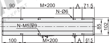
A向视图
