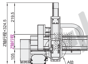
● A处放大图
