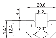
槽口详图
