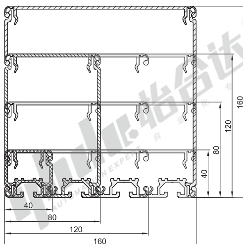
线槽型材组合示意图
