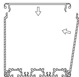
线槽型材组装图
