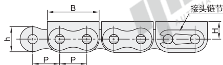
U型盖板链 VMT01/02
