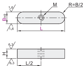
螺纹沉孔型
