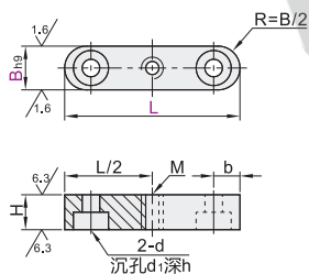
螺纹拆卸型
