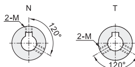
安装方式 (键槽+螺孔)
