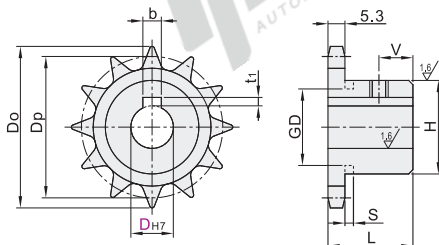
链轮 VLY01/02
