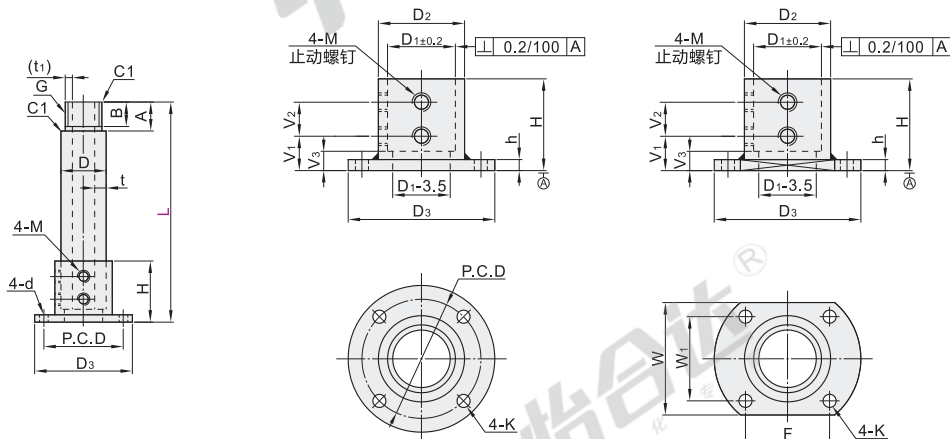
圆法兰型 RCB01/02/06
