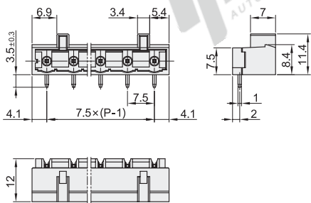
插头 ZKY17
