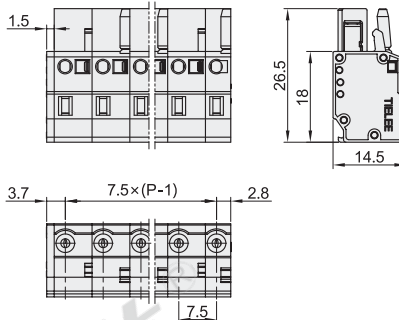
插座 ZKY18
