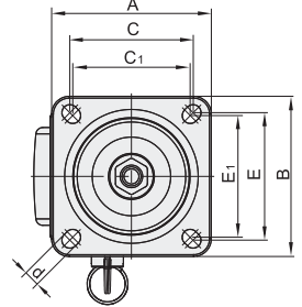
安装面 D60A/75A
