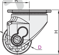
安装面 D60A/75A
