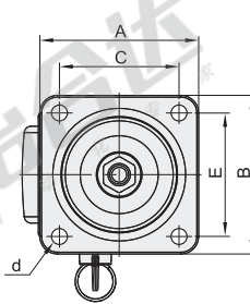
安装面 D60/75
