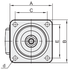
安装面 D60/75
