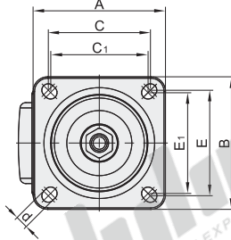
安装面 D60A/75A
