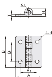
4孔安装
