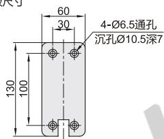
安装板尺寸
