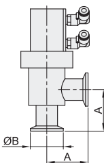
不带电磁阀 BLQ51
