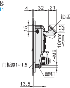
带锁芯 XAV18 无锁芯 XAV19
