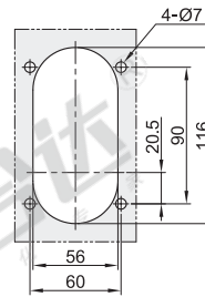
开孔尺寸
