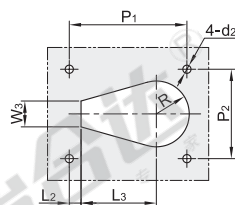
开孔尺寸(内装)
