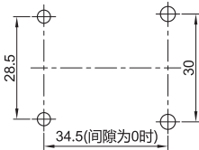
安装孔孔距
