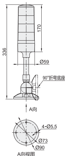
安装方式：A(可折式)
