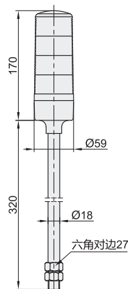
安装方式：E(螺杆式)
