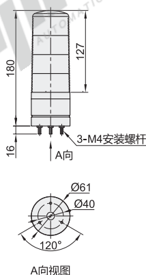
安装方式：C(直接安装式)
