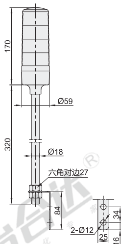
安装方式：L(L形支架式)
