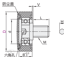
内六角外螺纹型(带防尘盖) E-BKR23
