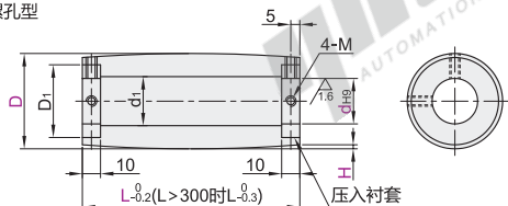
带肋槽直柱型 ENF21/26/31
