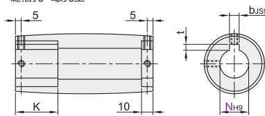
键槽+螺孔型
