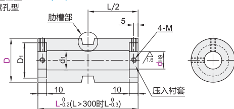
带肋槽直柱型 ENF21/26/31
