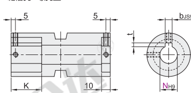
键槽+螺孔型
