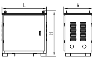
■ 防护式 (SBK-10kVA~60kVA)
