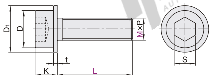
法兰型 TAC71
