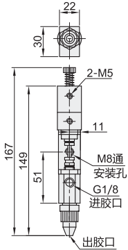
装配示意图
