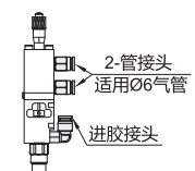
装配示意图
