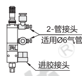
装配示意图
