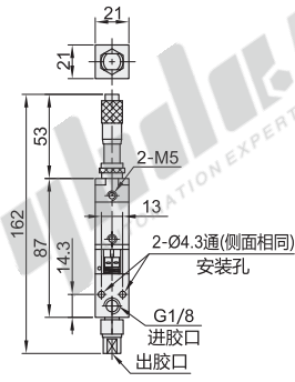
装配示意图
