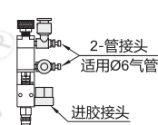
装配示意图
