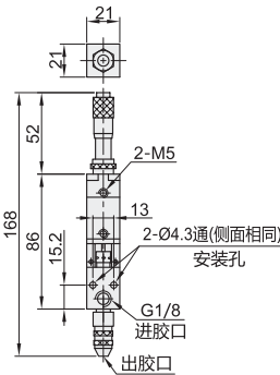
装配示意图
