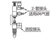
装配示意图
