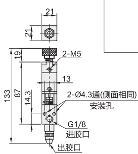
BMD50-03
