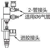
BMD50-06
