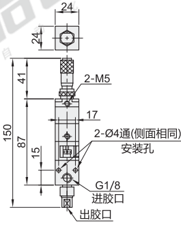
装配示意图
