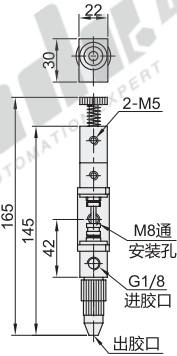
装配示意图
