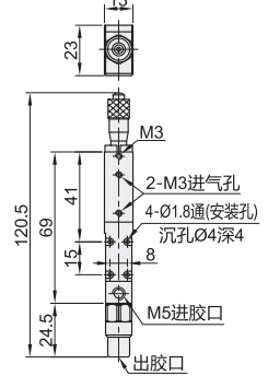
装配示意图
