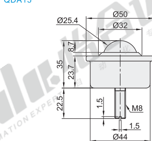
带一字槽螺栓型
