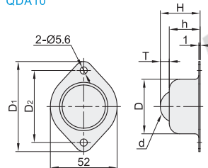
中载型·无垃圾排出孔
