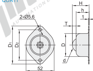
中载型·有垃圾排出孔
