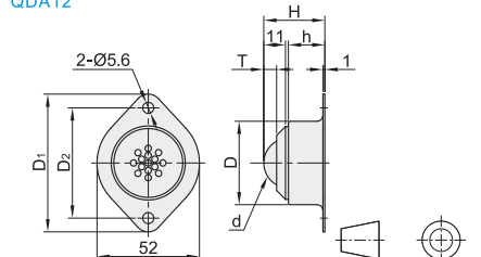
重载型·有垃圾排出孔
