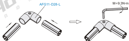
分解图
