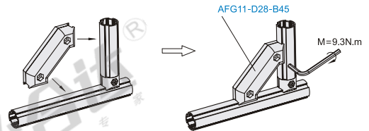
分解图
