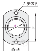
对边法兰型 Y-GVD21
