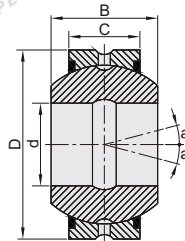
GEG...ES-2RS
