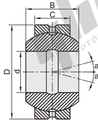
GEG...ES
