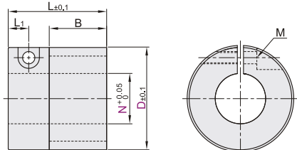
螺钉夹紧型 VNZ06
