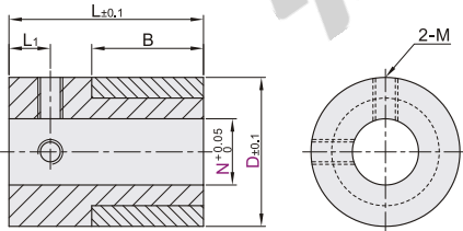
螺钉固定型 VNZ01
