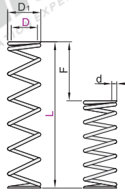
YNWL/J-YNWL 允许位移量 F_{max}=L \times 40\%
