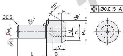
圆型 YDE21/22
