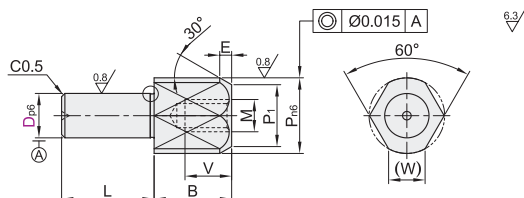
多棱型 YDE31/32
