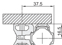
垫条+木螺钉装配方式
