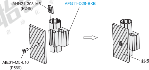
分解图
