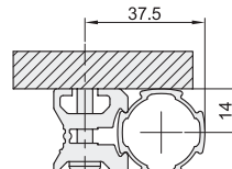
无垫条+木螺钉装配方式
