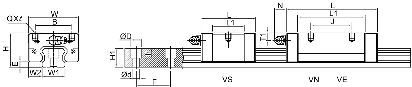
TRS-V 低組裝系列規格尺寸表
