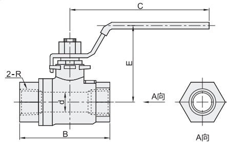
双片式大流量型 XZL96
