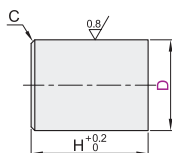
圆柱型 TFC52
