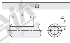
出力轴形状图
