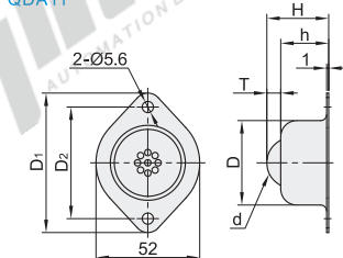
中载型·有垃圾排出孔 QDA11
