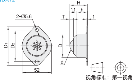
重载型·有垃圾排出孔 QDA12
