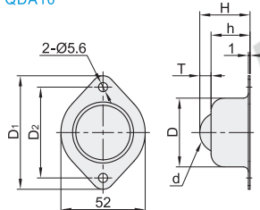
中载型·无垃圾排出孔 QDA10
