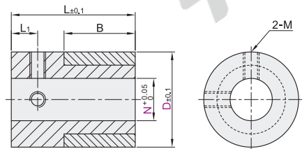
螺钉固定型 VNZ01
