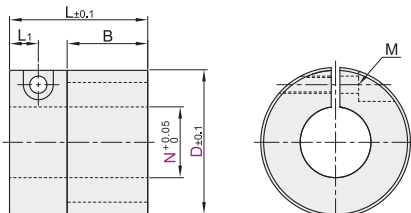
螺钉夹紧型 VNZ06
