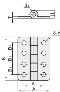
8孔安装
