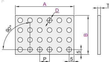
圆孔并列型(孔不可切断式) BLL08/09
