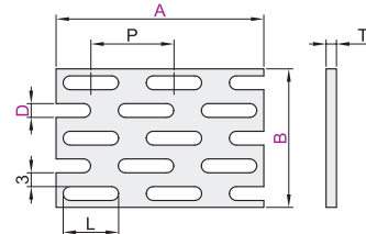
腰孔型 BLL10/15
