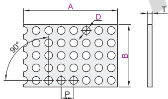
圆孔并列型(孔可切断式) BLL06/07
