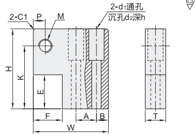
旗型限位块(螺纹孔) ICR34/35
