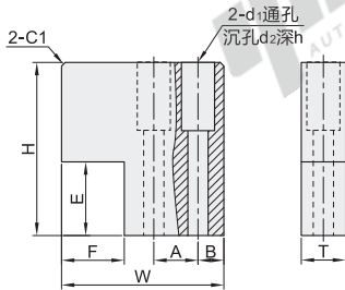
旗型限位块(无孔) ICR31
