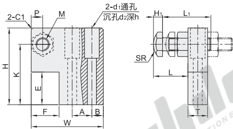
旗型限位块+定位螺栓 ICR41
