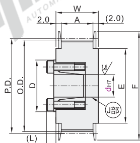
带轮形状
