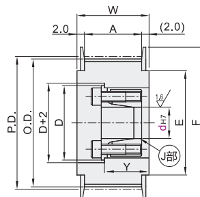
带轮形状
