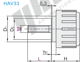
外螺纹型
