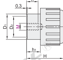
内螺纹型
