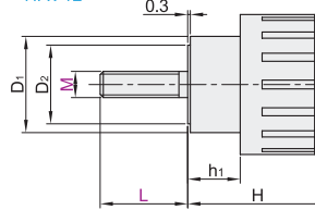
外螺纹型
