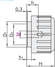
内螺纹型
