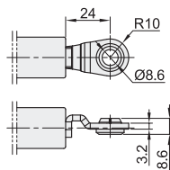
前端形状M
